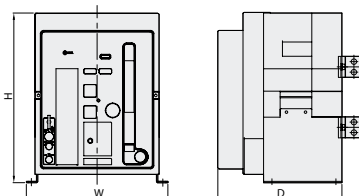
Стационарный тип
