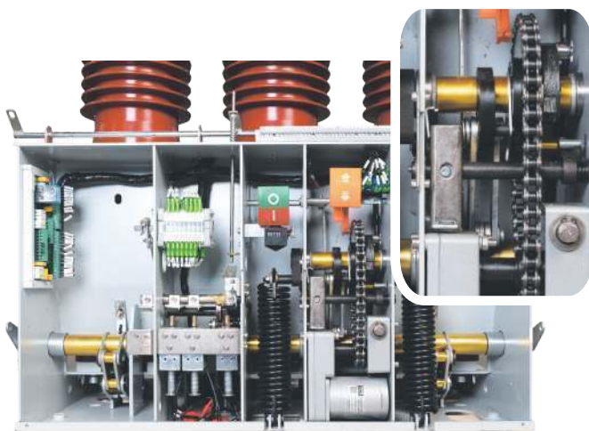
РИСУНОК 4-1. ВЫКЛЮЧАТЕЛЬ С ЦЕПНЫМ ИСПОЛНЕНИЕМ ПРИВОДА
