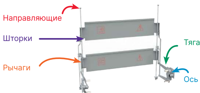
РИСУНОК 12. ШТОРОЧНЫЙ МЕХАНИЗМ
