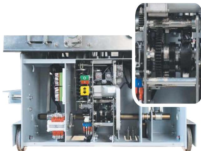
РИСУНОК 4-2. С МОДУЛЬНЫМ ИСПОЛНЕНИЕМ ПРИВОДА
