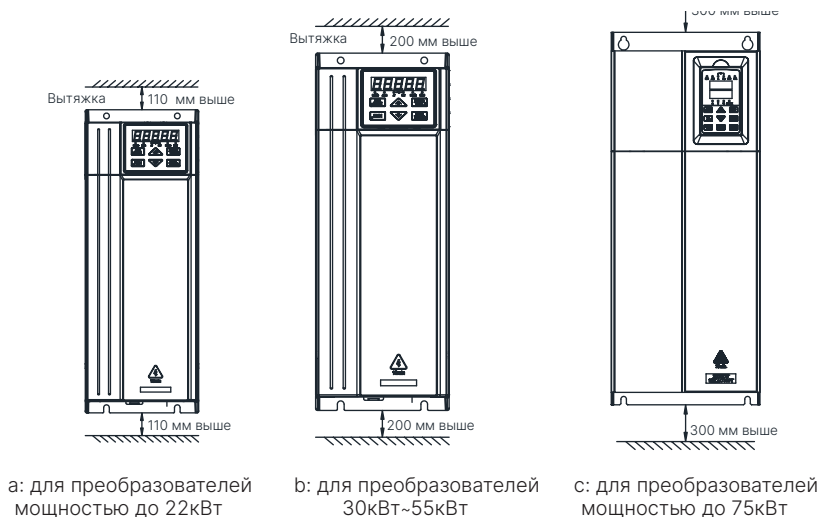
Рис. 3-1 Монтажные размеры
