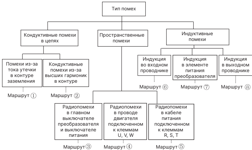
Рис.4-1 Типы помех
