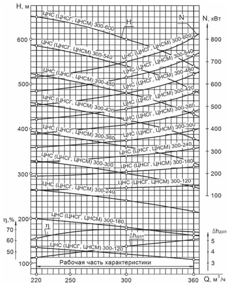
Рис.1.5 Характеристики насосов ЦНС (ЦНСГ, ЦНСМ)300-120...600
