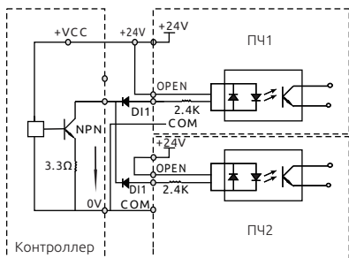
Рисунок 3-27. Параллельное подключение дискретных выходов разных ПЧ.
